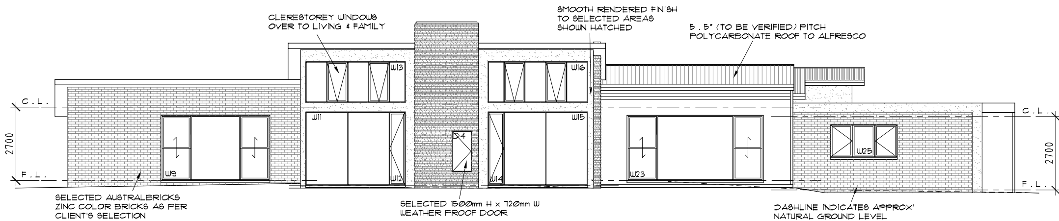
S O U T H S I D E E L E V A T I O N " 2 " 1 : 1 0 0
